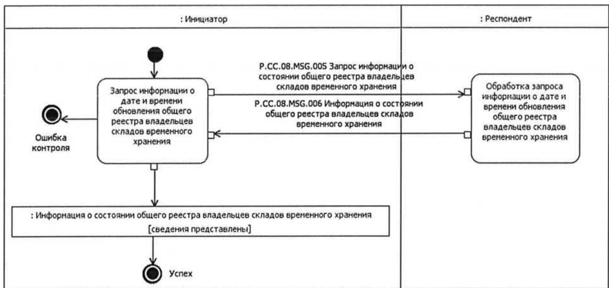
Рис. 7. Схема выполнения транзакции общего процесса «Получение информации о дате и времени обновления общего реестра владельцев складов временного хранения»
