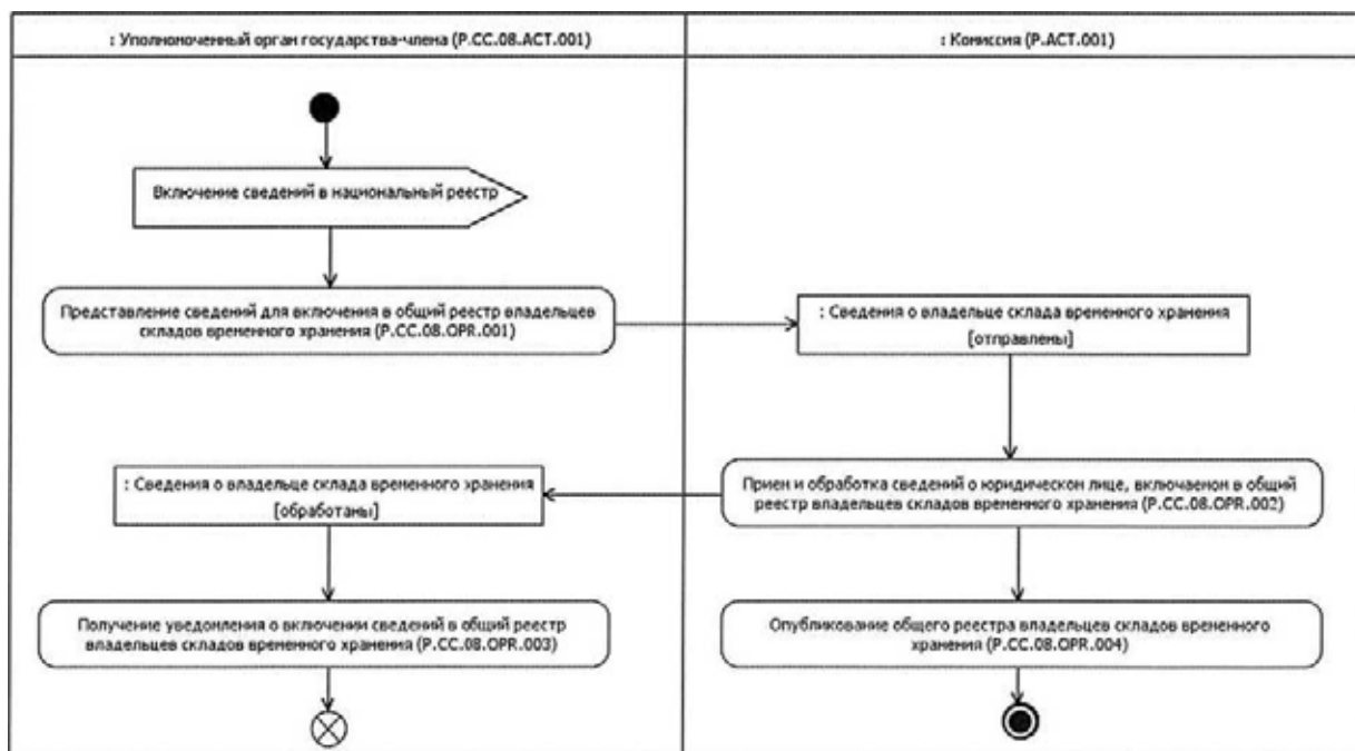
Рис. 5. Схема выполнения процедуры «Включение сведений в общий реестр владельцев складов временного хранения» (P.CC.08.PRC.001)
