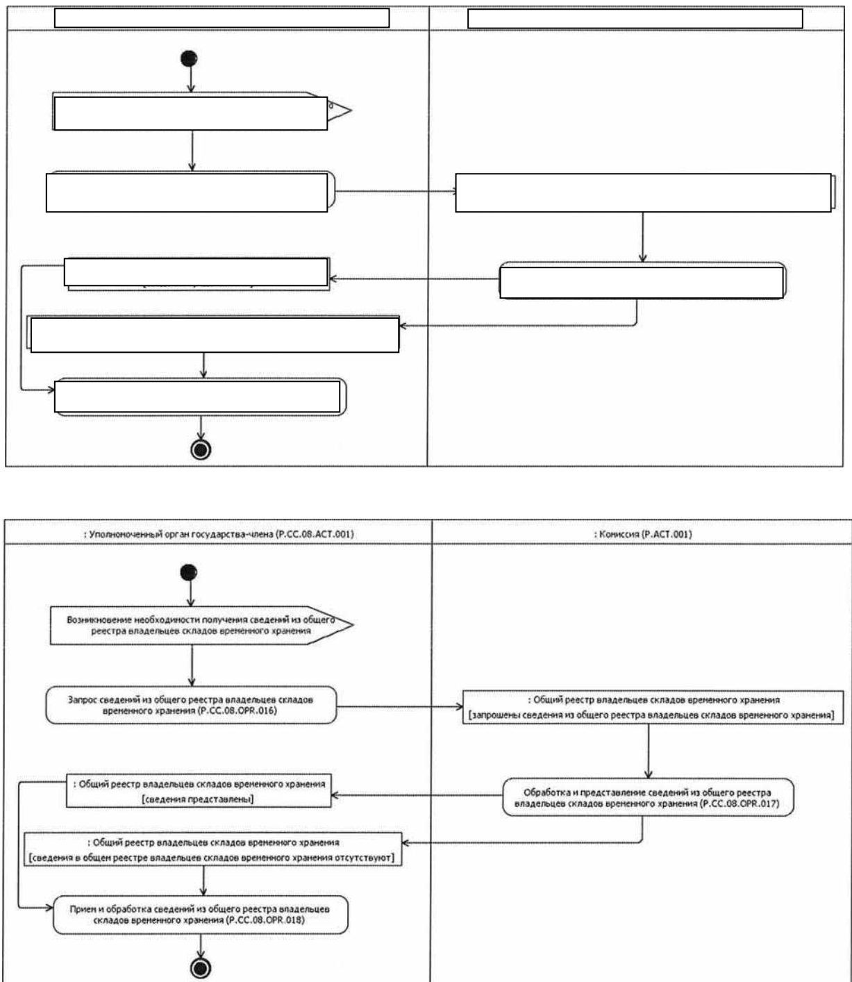
Рис. 9. Схема выполнения процедуры «Получение сведений из общего реестра владельцев складов временного хранения» (P.CC.08.PRC.005)
