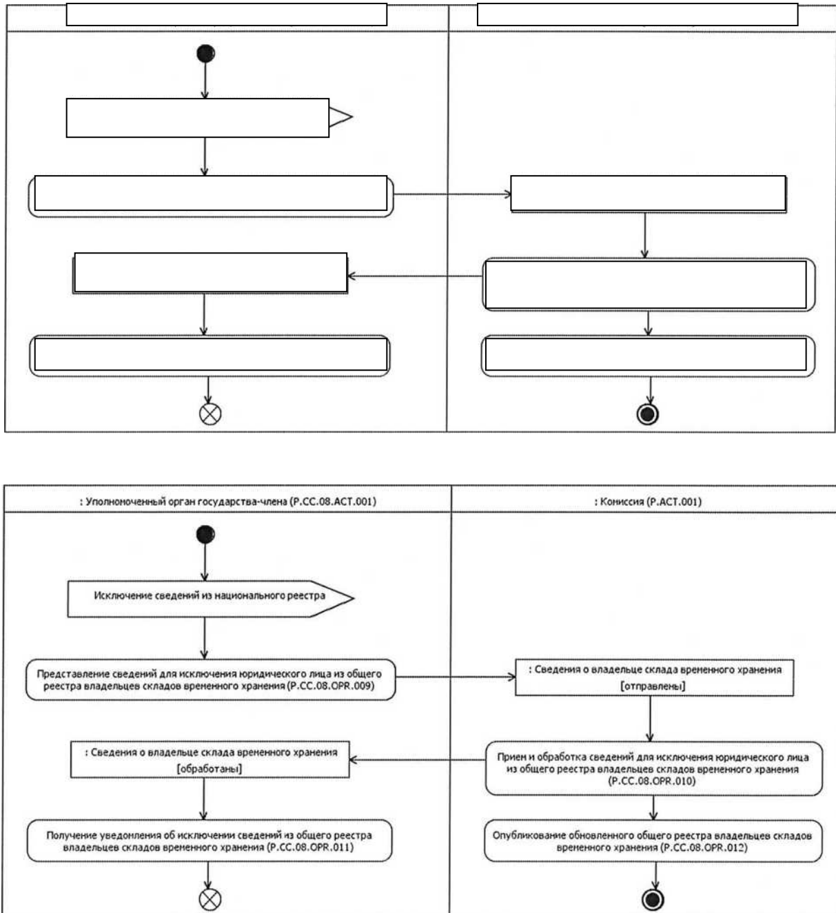
Рис. 7. Схема выполнения процедуры «Исключение сведений из общего реестра владельцев складов временного хранения» (P.CC.08.PRC.003)
