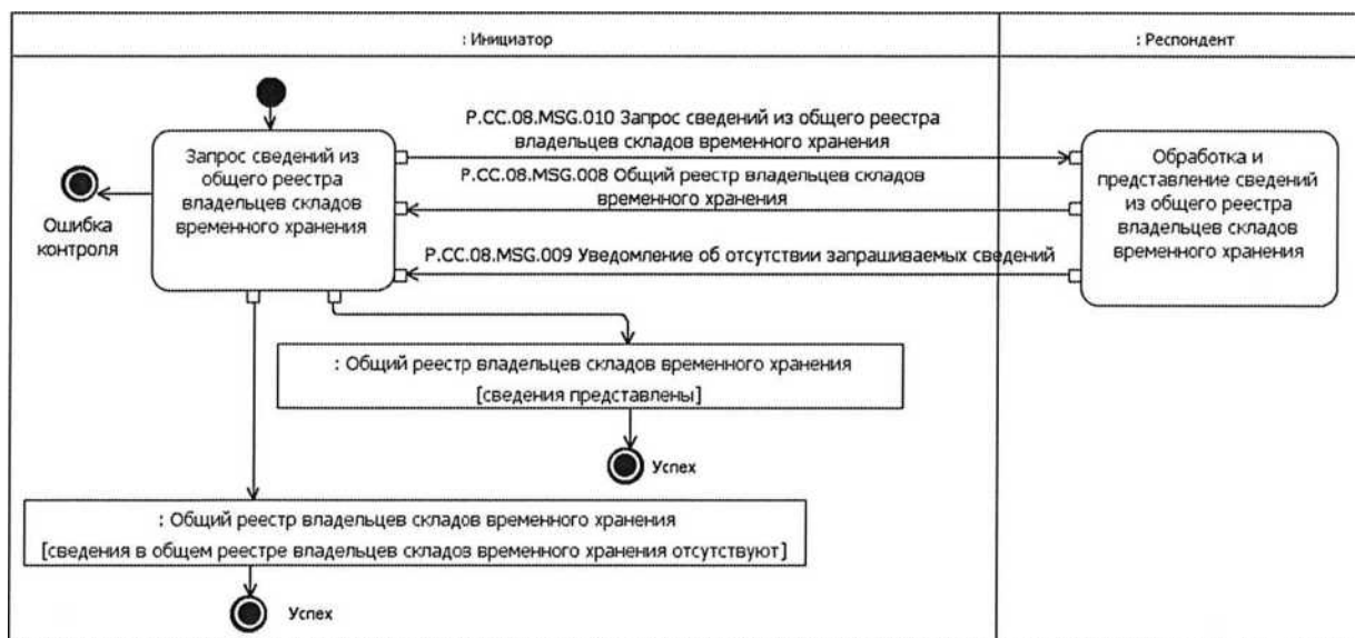
Рис. 8. Схема выполнения транзакции общего процесса «Получение сведений из общего реестра владельцев складов временного хранения» (P.СC.08.TRN.005)
