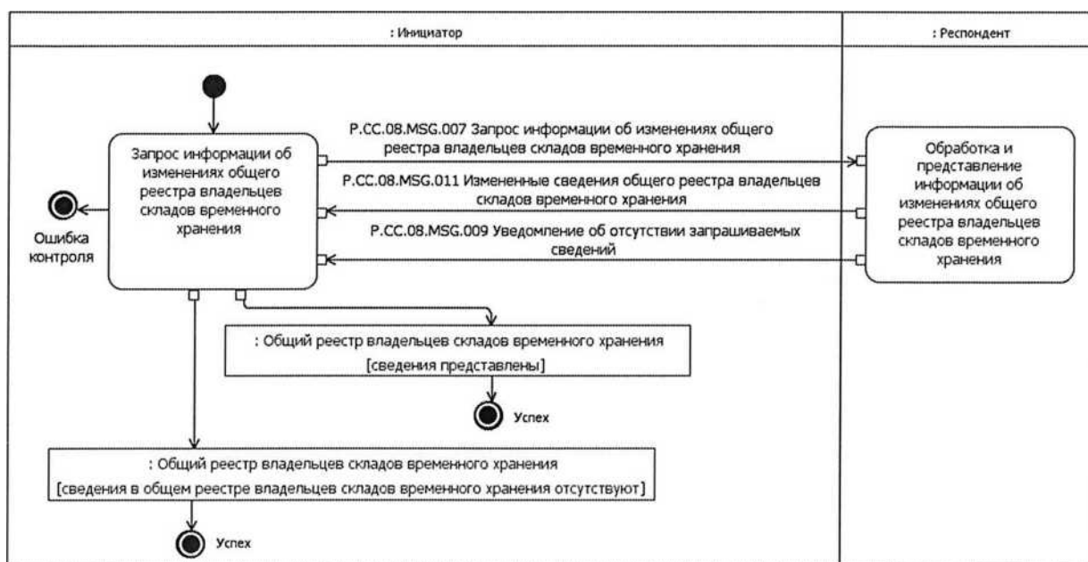
Рис. 9. Схема выполнения транзакции общего процесса «Получение информации об изменениях, внесенных в общий реестр владельцев складов временного хранения»
