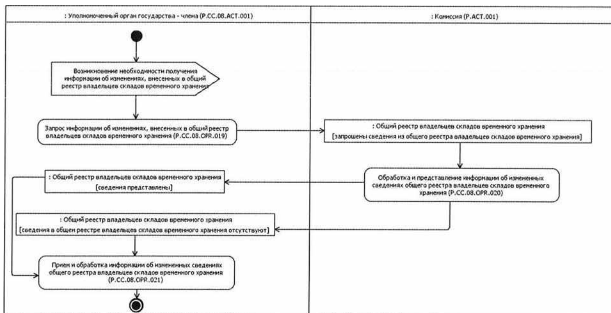
Рис. 10. Схема выполнения процедуры «Получение информации об изменениях, внесенных в общий реестр владельцев складов временного хранения» (P.CC.08.PRC.006)
