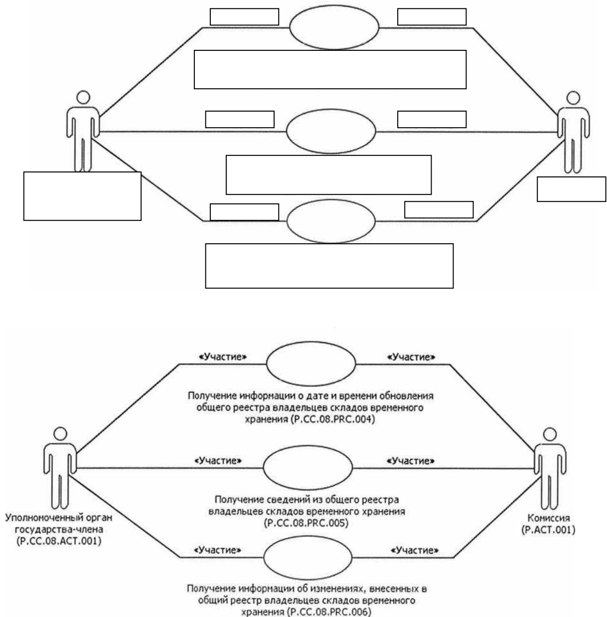
Рис. 3. Общая схема выполнения группы процедур представления уполномоченным органам государств-членов сведений, содержащихся в общем реестре владельцев складов временного хранения
