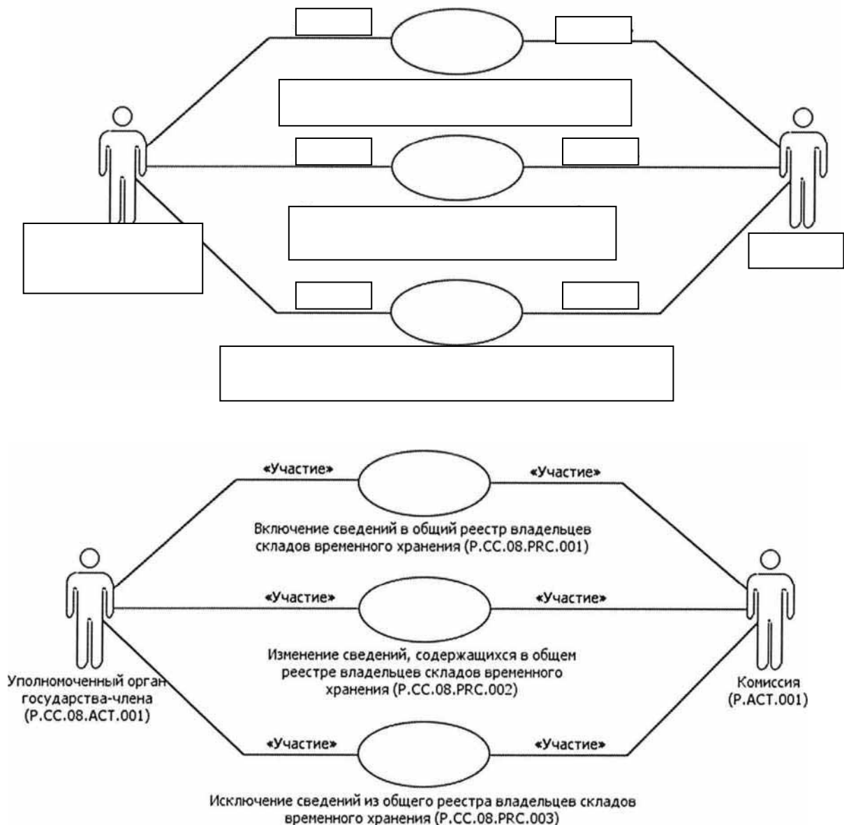
Рис. 2. Общая схема выполнения группы процедур формирования и ведения общего реестра владельцев складов временного хранения
