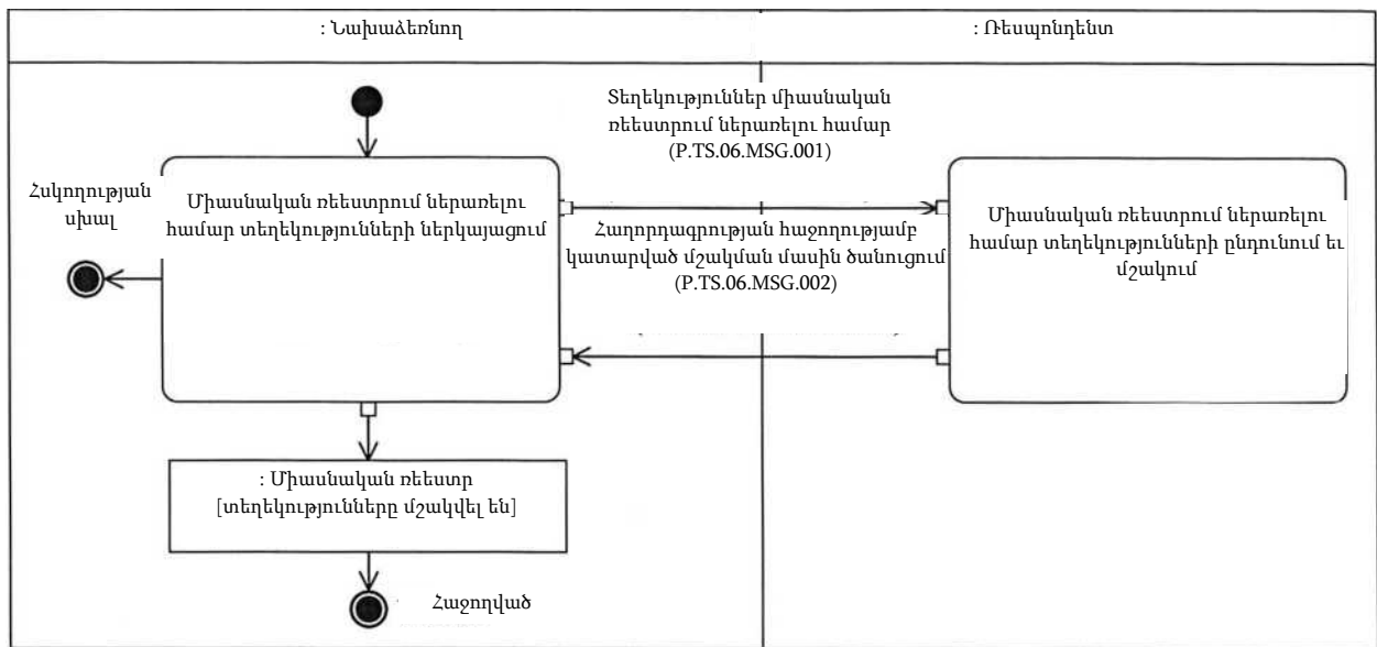
Նկ. 4. «Միասնական ռեեստրում տեղեկությունների ներառում» ընդհանուր գործընթացի տրանզակցիայի (P.TS.06.TRN.001) կատարման սխեման
