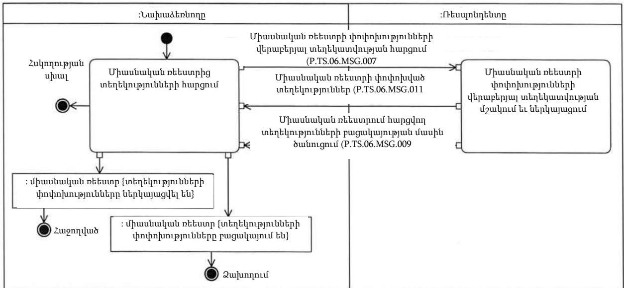
Նկ. 5. «Միասնական ռեեստրում կատարված փոփոխությունների վերաբերյալ տեղեկատվության ստացում» ընդհանուր գործընթացի տրանզակցիայի (P.TS.06.TRN.006) կատարման սխեմա
