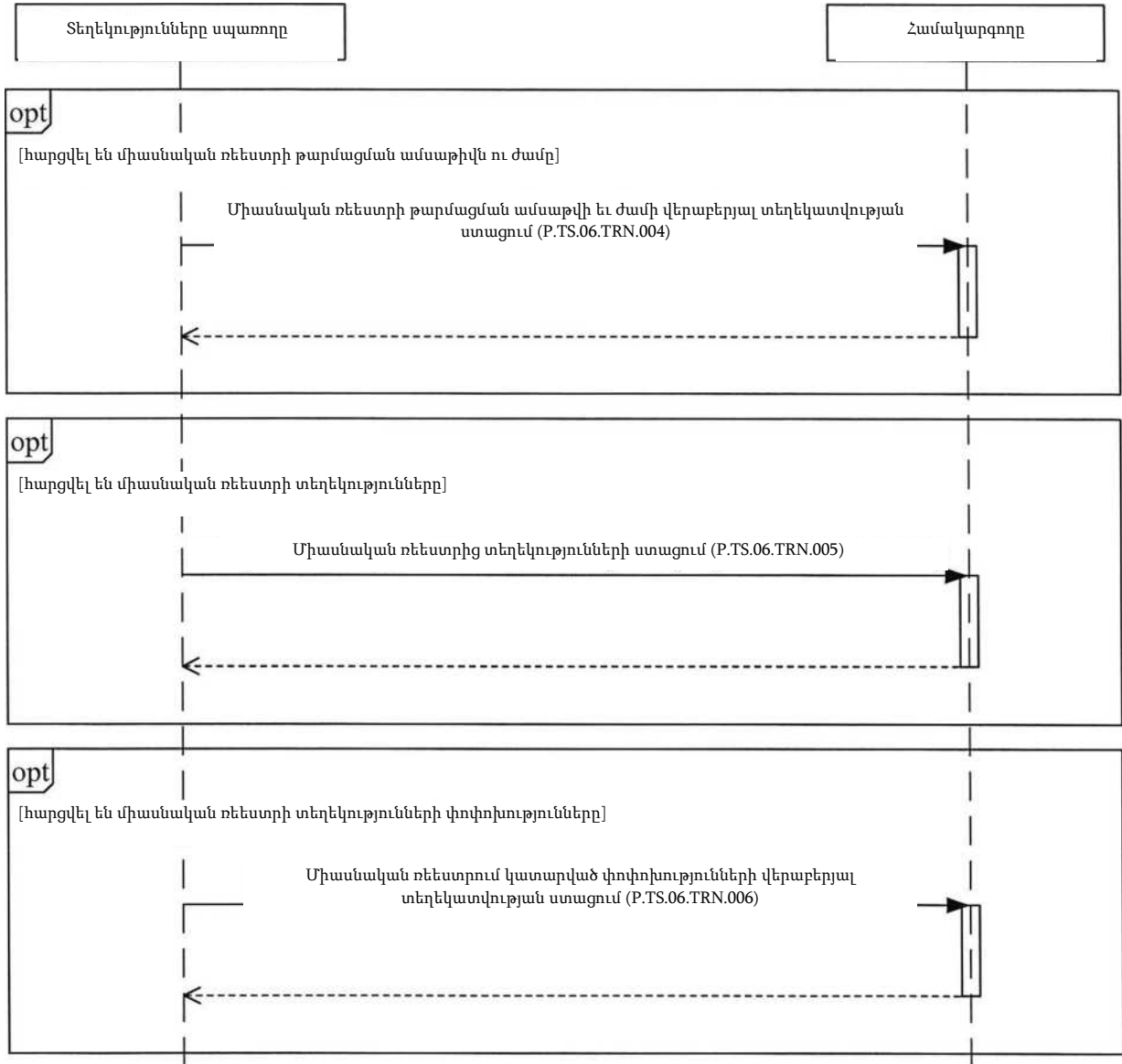
Նկ. 2. Միասնական ռեեստրում պարունակվող տեղեկություններն էլեկտրոնային անձնագրերի համակարգերի վարիչին ներկայացնելիս ընդհանուր գործընթացի տրանզակցիաների կատարման սխեմա
