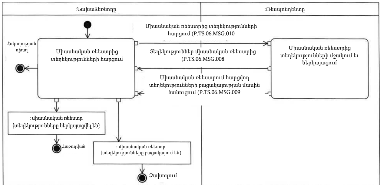
Նկ. 4. «Միասնական ռեեստրից տեղեկությունների ստացում» ընդհանուր գործընթացի տրանզակցիայի (P.TS.06.TRN.005) կատարման սխեմա
