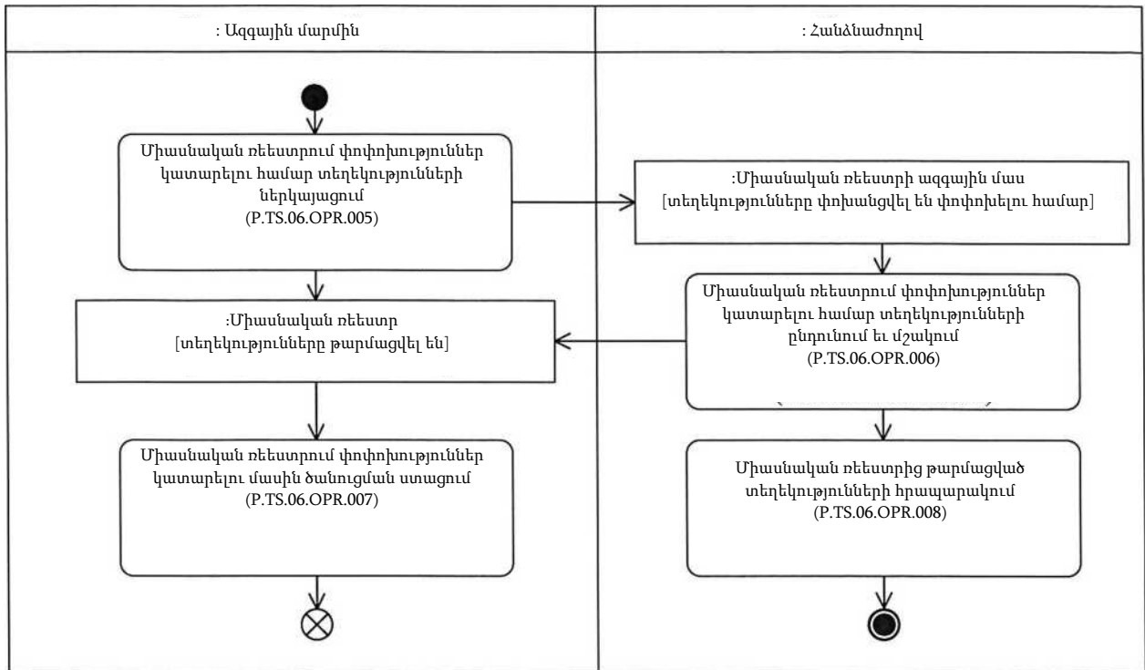
Նկ. 6. «Միասնական ռեեստրում պարունակվող տեղեկությունների փոփոխում» ընթացակարգի (P.TS.06.PRC.002) կատարման սխեման
