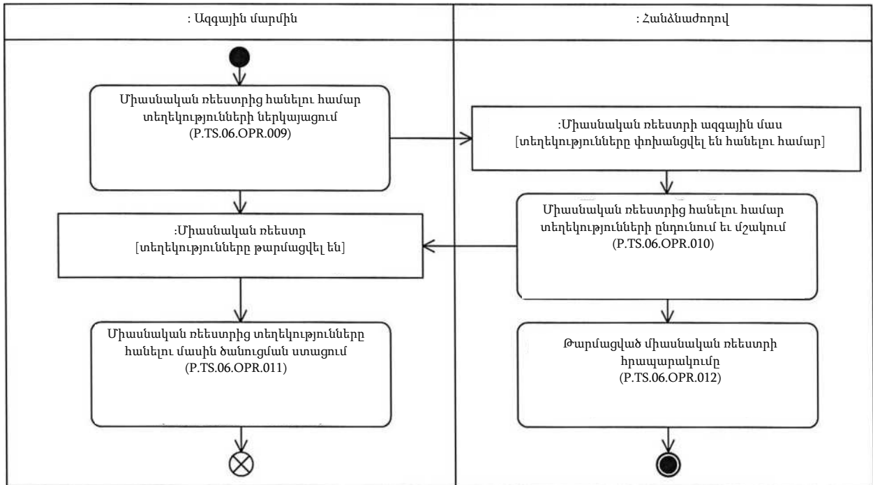
Նկ. 7. «Միասնական ռեեստրից տեղեկությունների հանում» ընթացակարգի (P.TS.06.PRC.003) կատարման սխեման
