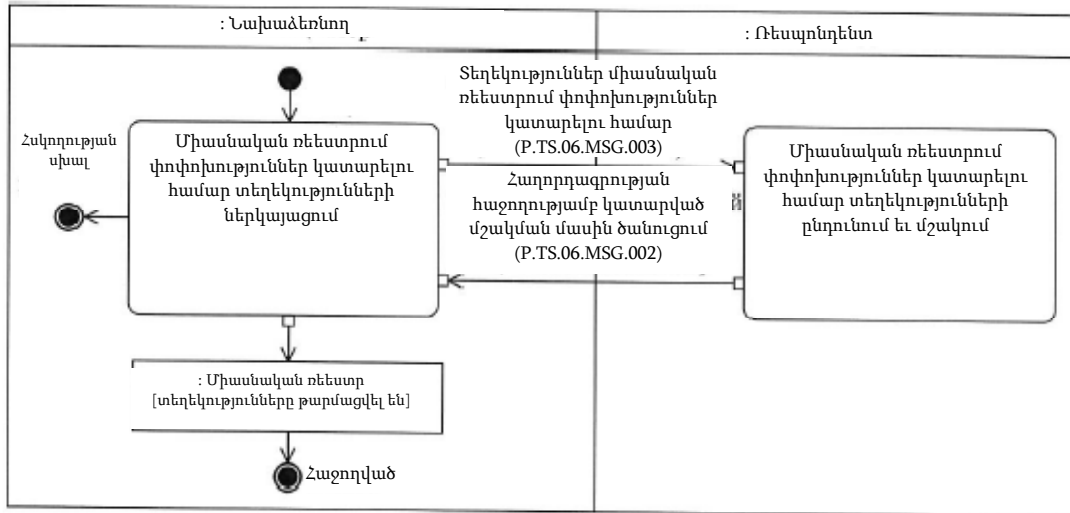
Նկ. 5. «Միասնական ռեեստրի տեղեկությունների փոփոխում» ընդհանուր գործընթացի տրանզակցիայի (P.TS.06.TRN.002) կատարման սխեմա
