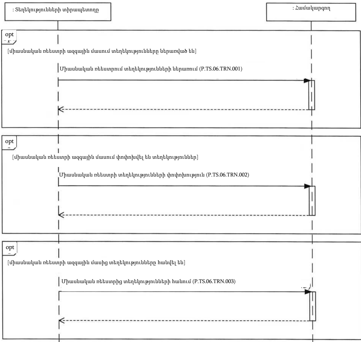
Նկ. 2. Ընդհանուր գործընթացի տրանզակցիաների կատարման սխեման՝ միասնական ռեեստրը ձեւավորելիս եւ վարելիս
