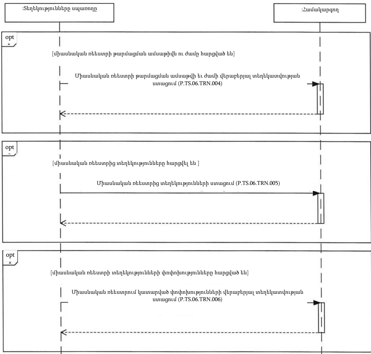
Նկ. 3. Միասնական ռեեստրում պարունակվող տեղեկություններն ազգային մարմիններ ներկայացնելիս ընդհանուր գործընթացի տրանզակցիաների կատարման սխեմա
