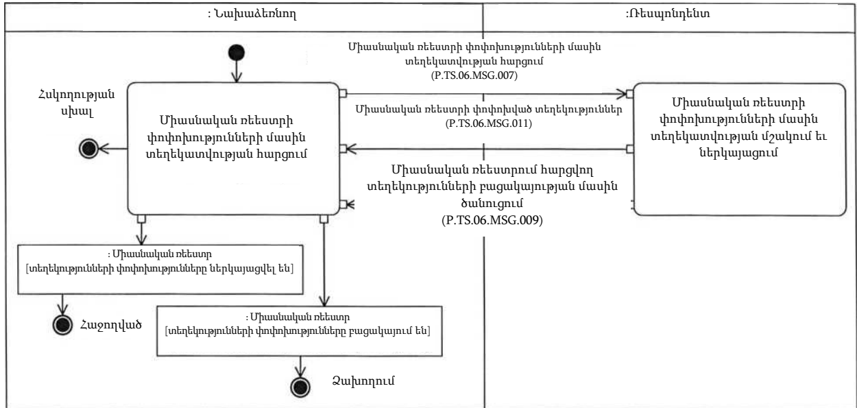
Նկ. 9. «Միասնական ռեեստրում կատարված փոփոխությունների մասին տեղեկատվության ստացում» ընդհանուր գործընթացի տրանզակցիայի (P.TS.06.TRN.006) կատարման սխեման
