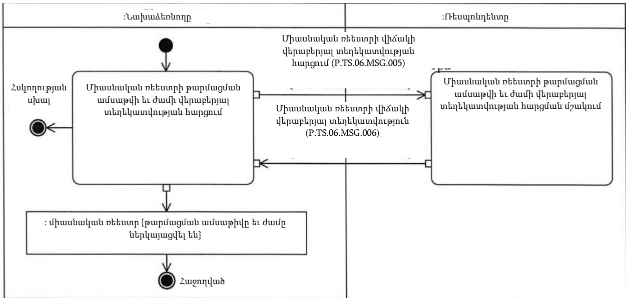
Նկ. 3. «Միասնական ռեեստրի թարմացման ամսաթվի եւ ժամի վերաբերյալ տեղեկատվության ստացում» ընդհանուր գործընթացի տրանզակցիայի (P.TS.06.TRN.004) կատարման սխեմա
