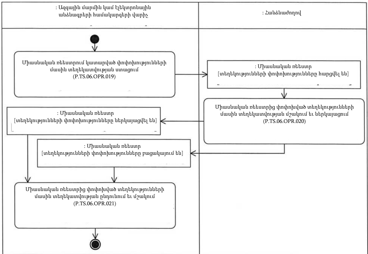
Նկ. 10. «Միասնական ռեեստրում կատարված փոփոխությունների մասին տեղեկատվության ստացում» ընթացակարգի (P.TS.06.PRC.006) կատարման սխեման
