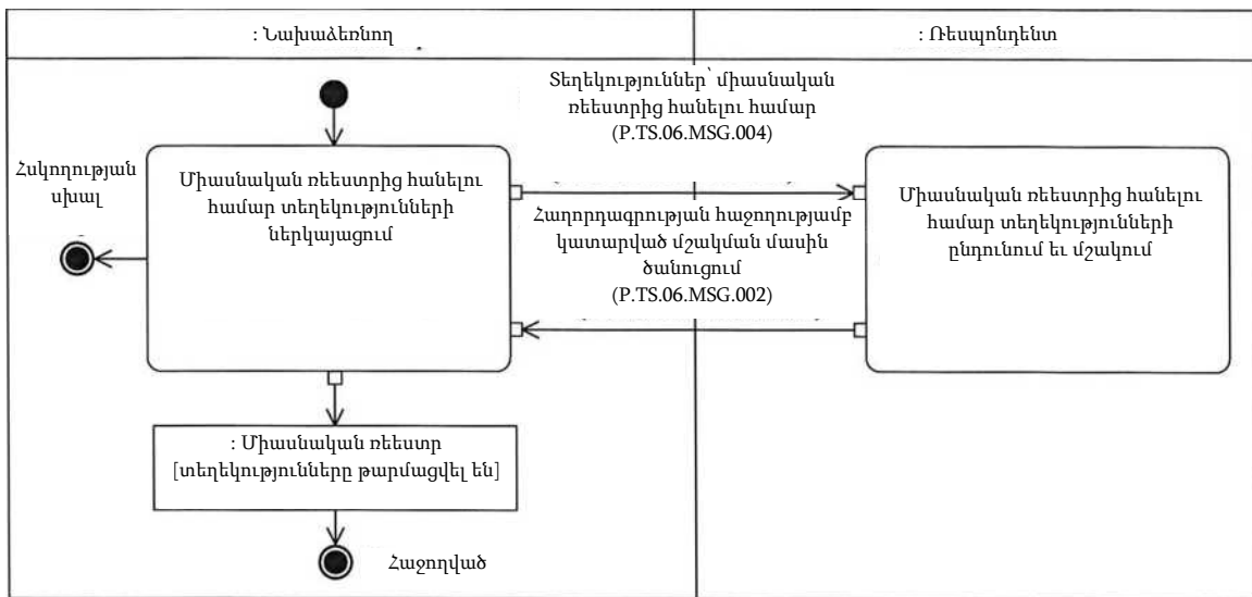
Նկ. 6. «Միասնական ռեեստրից տեղեկությունների հանում» ընդհանուր գործընթացի տրանզակցիայի (P.TS.06.TRN.003) կատարման սխեման
