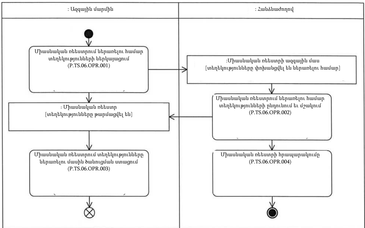
Նկ. 5. «Միասնական ռեեստրում տեղեկությունների ներառում» ընթացակարգի (P.TS.06.PRC.001) կատարման սխեման
