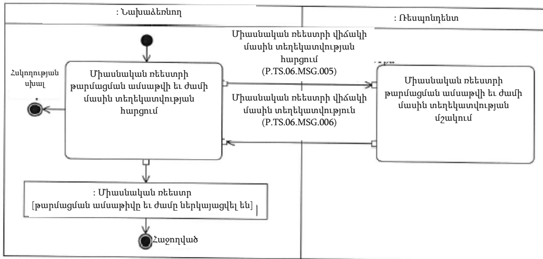
Նկ. 7. «Միասնական ռեեստրի թարմացման ամսաթվի եւ ժամի մասին տեղեկատվության ստացում» ընդհանուր գործընթացի տրանզակցիայի (P.TS.06.TRN.004) կատարման սխեման
